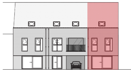
Achtergevel
