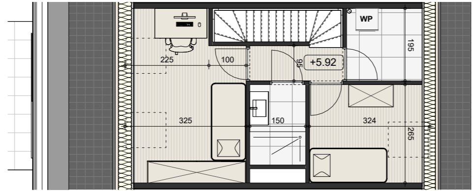
Verdieping +2
