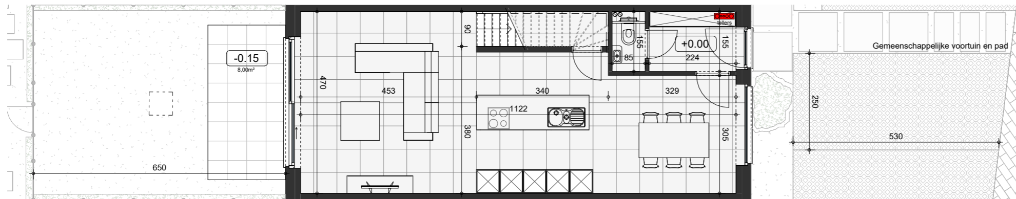
Gelijkvloers
