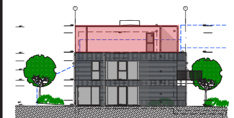
Zijgevel links
