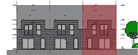
Achtergevel
